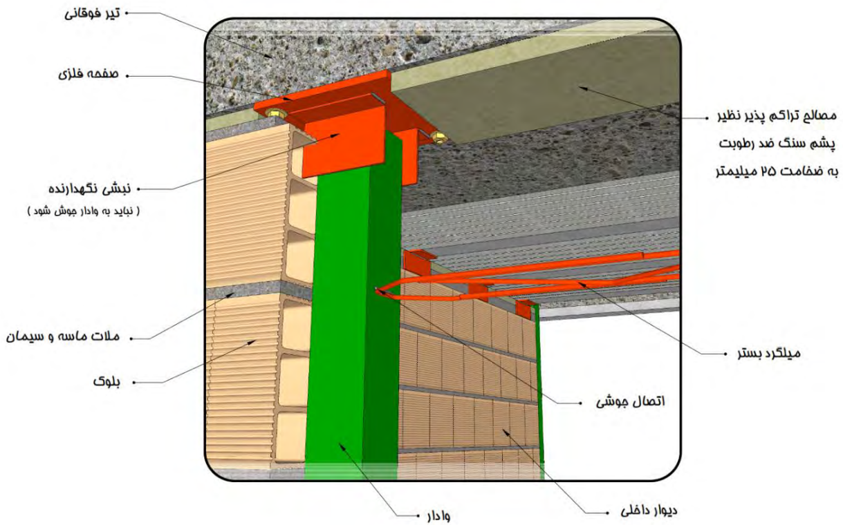
الف- به صورت اتصال کشویی با استفاده از نیشی
