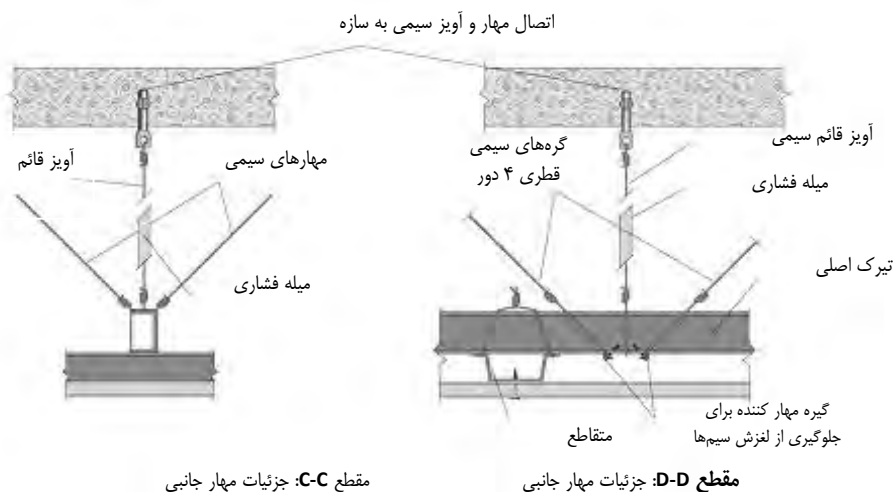
شکل پ-۳۴- جزئیات مهاربندی جانبی برای سقف پانل گچی معلق مقاطع نشان داده شده در شکل پ-۳۶-۲۸
