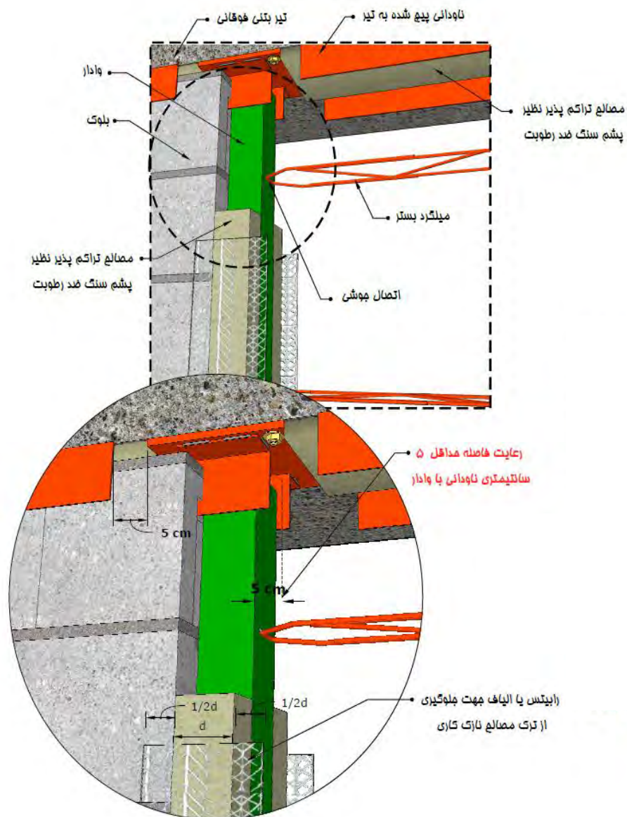
شکل پ ۴-۶-۴- اجرای عایق پشم سنگ و مش الیاف یا رابطیس بر روی وادر
