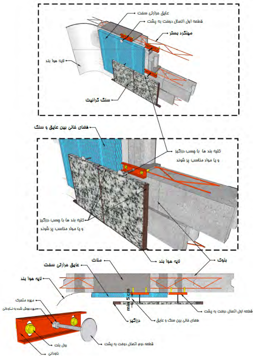
ب- نمونه ای از اجرای دوخت به پشت نمای سنگی به دیوار در محل مسلح سازی دیوار شکل ۶-۳۰- نمونه‌هایی از اجرای دوخت به پشت نمای سنگی به دیوار و جزئیات اجرایی آن
