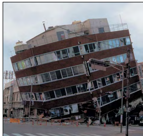
شکل ۳-۶- فاصله زیاد بین مرکز جرم و مرکز سختی و خرابی ناشی از ایجاد پیشش
