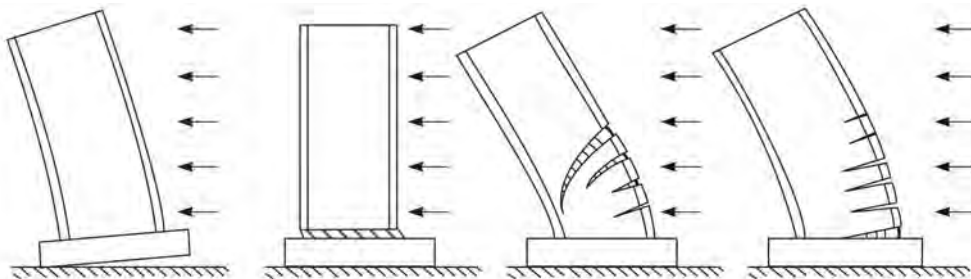
شکل ۳۱-۴ - انواع حالت‌های شکست دیوار برشی
