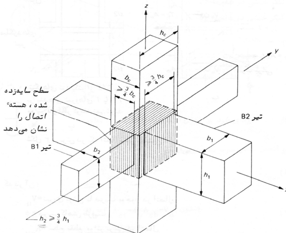
شکل ۱۷-۶-۲ هسته اتصال
