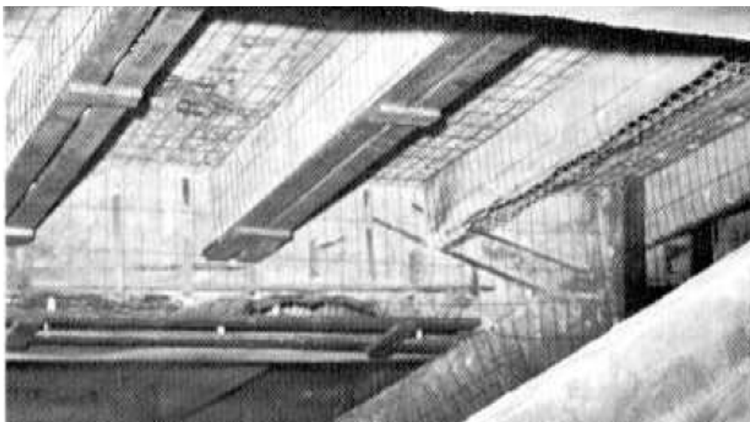
شکل ۲-۳-۳- افزایش ضخامت دال از قسمت تحتانی با شاکریت
