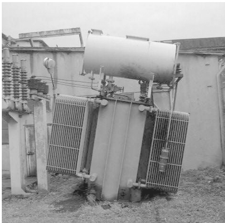
شکل ۱۰-۱۲ - آسیب وارده به میدل برق
