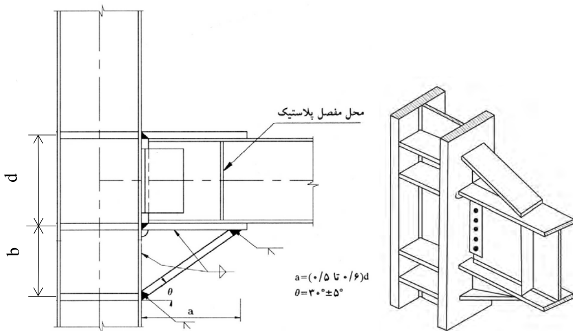
شکل ۲-۶-۲ جزئیات ماهیچه تحتانی برای تقویت اتصال
