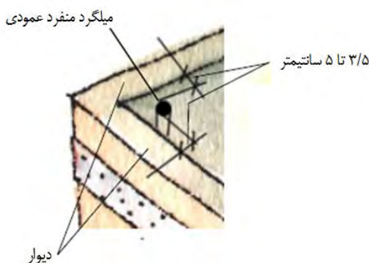
شکل ۹-۲۰ میلگردهای قائم اصلی باید حداقل 3/5 تا 5 سانتیمتر از دیوار فاصله داشته باشد
