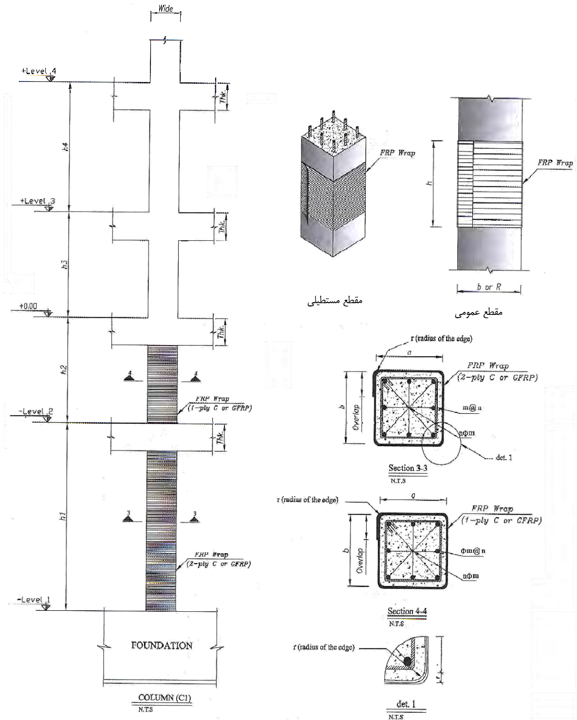
شکل ۲-۵-۱۸- جزئیات تیپ بهسازی ستون‌های بتنی با مصالح FRP
