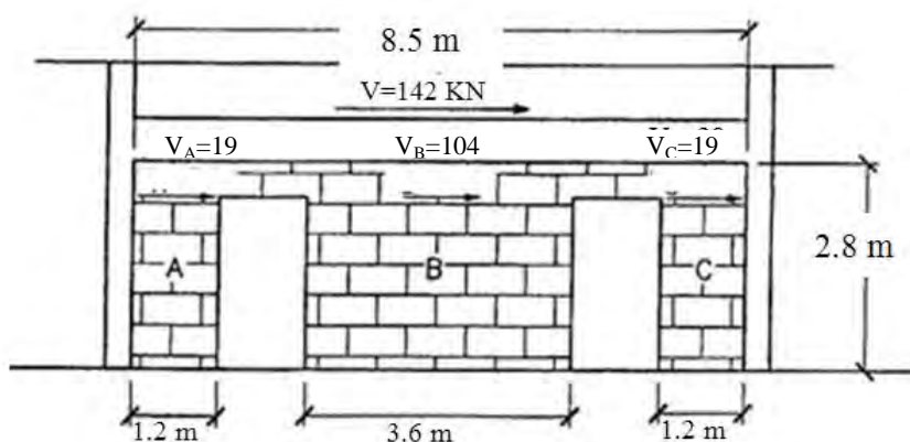
شکل مثال ۴-۲-ر- دیوار طولی طبقه همکف محور C
