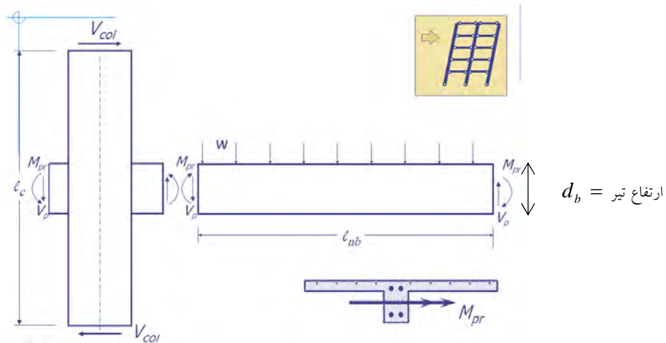
شکل ۶-۲-۱ نمایش محل تشکیل مفصل پلاستیک در تیر و فاصله آن از بر ستون
