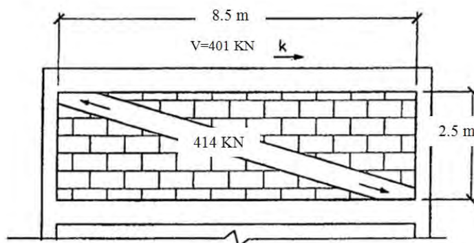
شکل مثال ۴-۲-ذ- دیوار طولی طبقه دوم محور D
