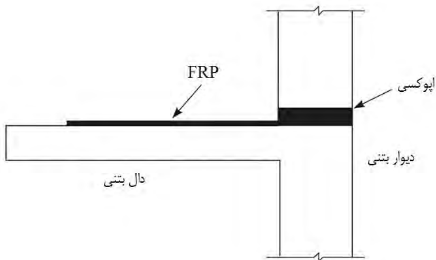
شکل ۱۳-۳-۲- تأمین طول مهاربندی با امتداد FRP در داخل اتصال
