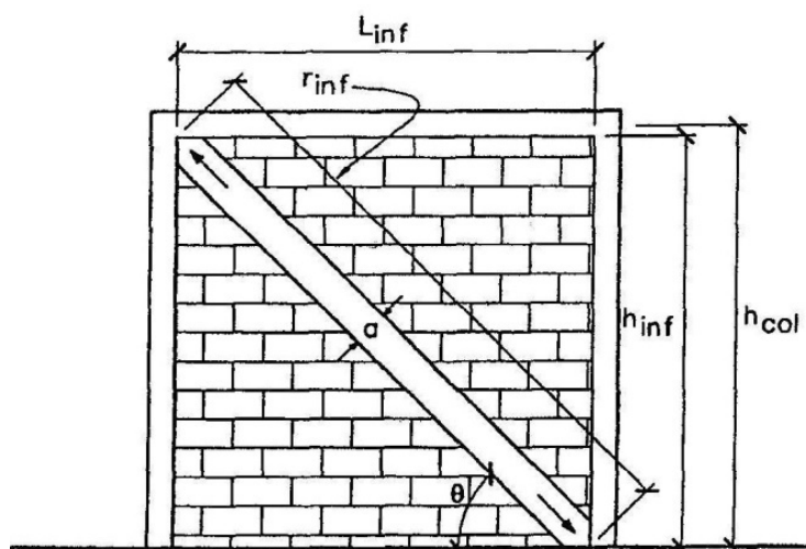
شکل مثال ۴-۲-ج تعریف پارامترهای دستک فشاری
