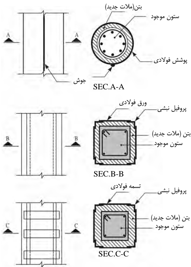
شکل ۲-۵-۱۰- استفاده از روکش فولادی در بهسازی ستونهای بتنی
