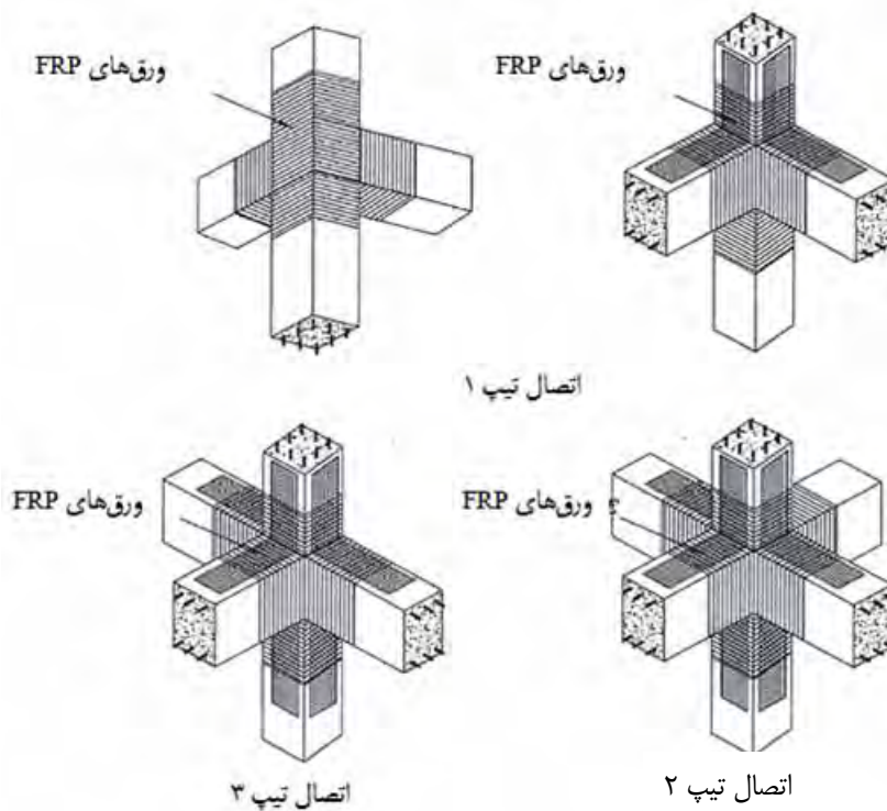
شکل ۲-۶-۳۰ جزئیات تیپ استفاده از FRP در مقاوم‌سازی اتصالات
