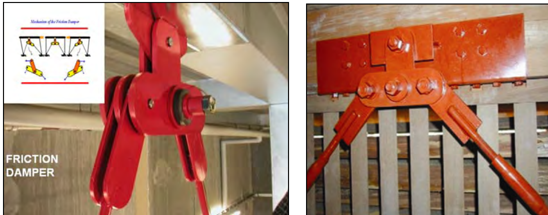
شکل ۷-۵- استفاده از میراگرهای اصطکاکی چرخشی در مقاوم سازی
