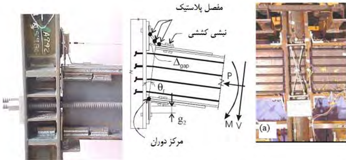
شکل ۲-۶-۴ مقاومت‌سازی اتصال با پیش‌تندگی خارجی بوسیله کابل کششی
