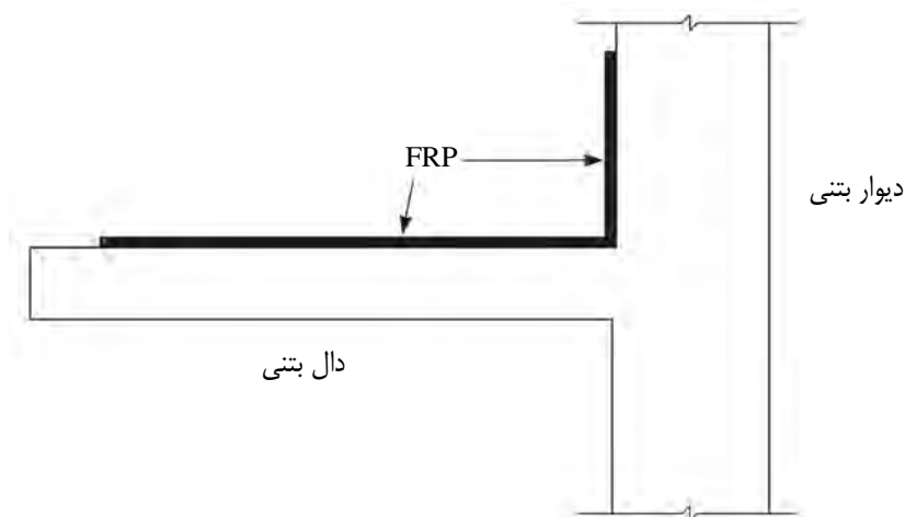
شکل ۱۲-۳-۲- تأمین طول مهاربندی با امتداد FRP به روی دیوار
