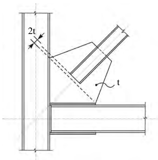
شکل ۴-۹- اتصال مهاربندی با ایجاد خط آزاد خمشی
