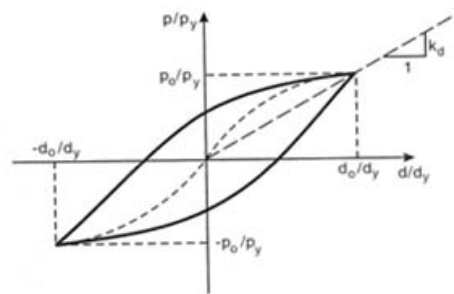
شکل ۷-۲۲- رفتار چرخه‌ای مدل‌های غیرخطی نیرو-تغییر مکان
