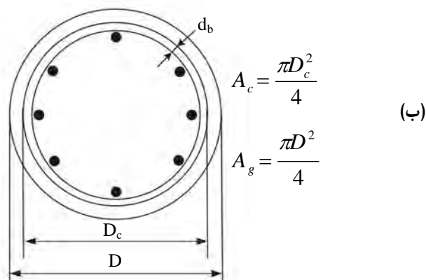
شکل ۲-۶-۱۸ شکل تنگ مستطیلی و مارپیچ برای ارتفاع S_h از هسته ستون
