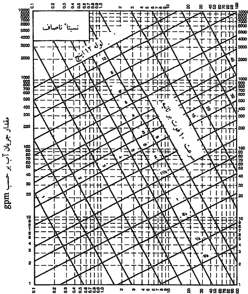
اقت فشار آب بر حسب فوت بر اینچ مربع در ۱۰۰ فوت طول
