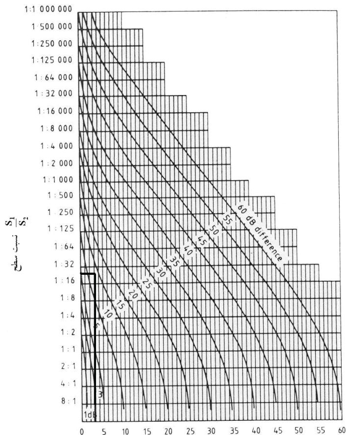
شکل پ-۲-۳: نمودار تخمین شاخص کاهش صدای جداکننده مرکب
