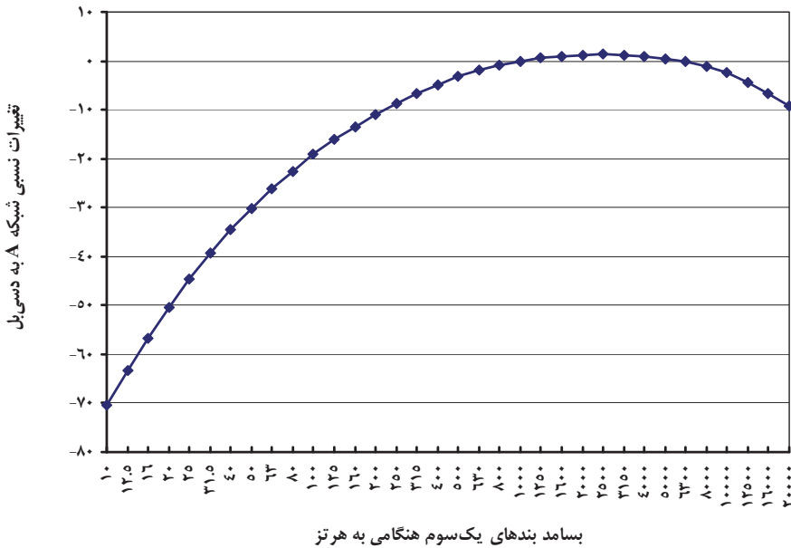
شکل ۱-۱۸-۳-۳: نمودار تغییرات نسبی شبکه وزنی A در بسامدهای مختلف
