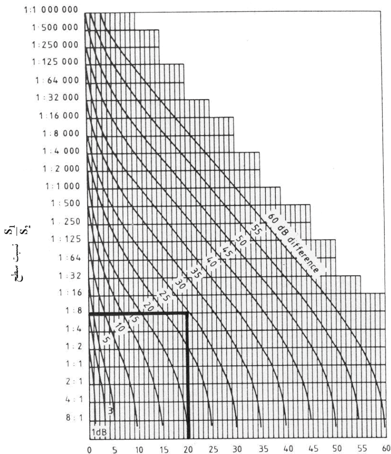
R_1-R_2 کسر شده از شاخص کاهش صدای بیشتر
