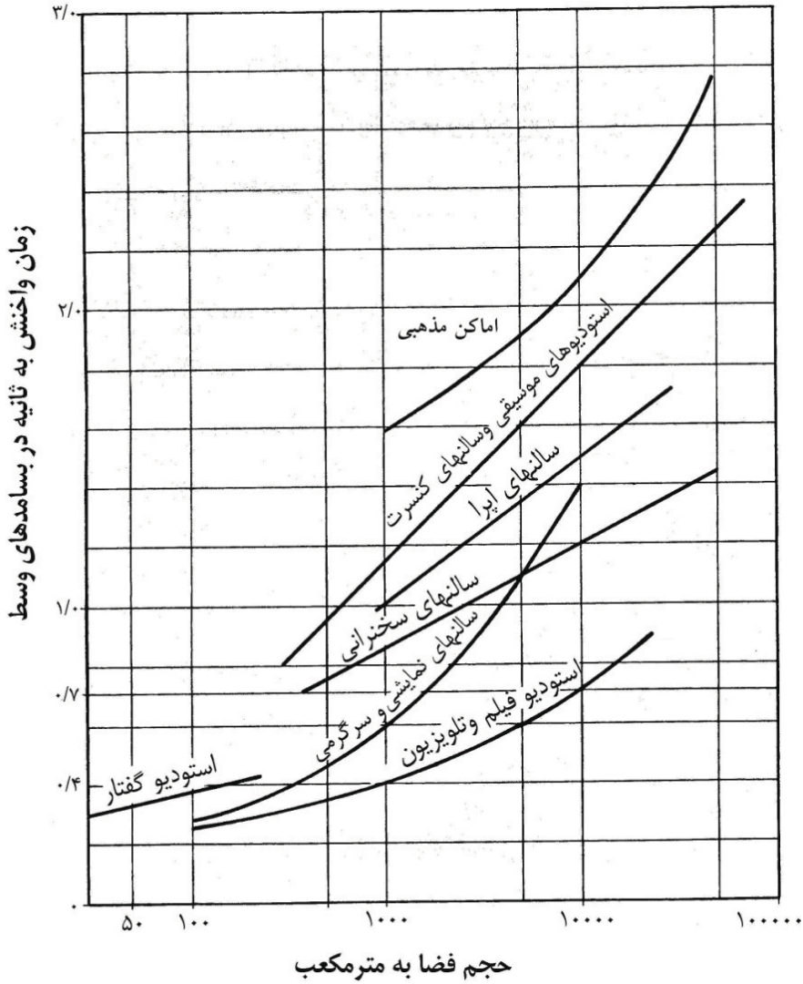
شکل ۱-۷-۲-۱۸: نمودار زمان واخنش بهینه در فضاهای مختلف
