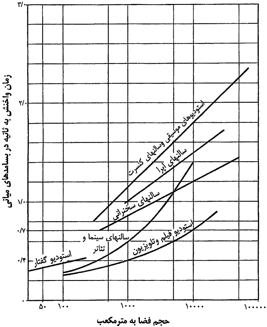
شکل ۱۸-۲-۱: نمودار زمان واخنش بهینه در فضاهای مختلف
