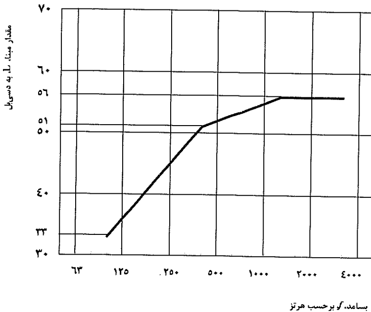
شکل ۱۸-۱-۳-۴: نمودار مقادیر مینا برای صدای هواپرد، در بندهای یک سوم هنگامی
