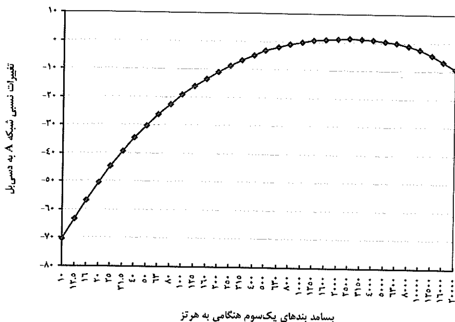
شکل ۱۸-۱-۳-۶: نمودار تغییرات نسبی شبکه وزنی A در بسامدهای مختلف
