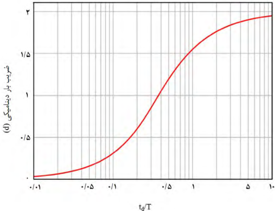
شکل ۲۱-۵-۶- ضریب بار دینامیکی برای انفجار با فاصله
